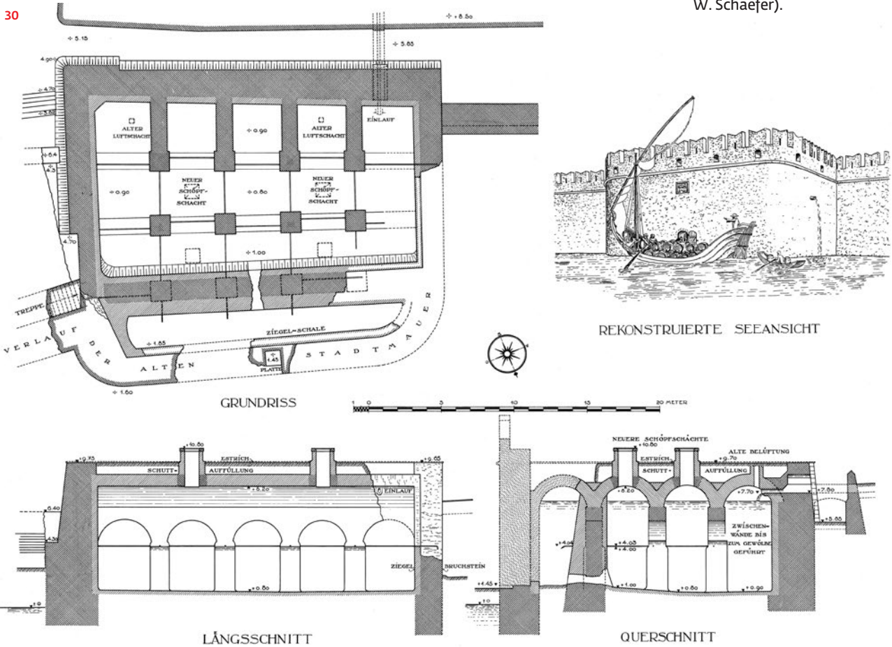
30 Η δεξαμενή του ενετικού λιμανιού. Σχεδιαστική αποτύπωση και αναπαράσταση του W. Schaefer (αρχείο W. Schaefer).
