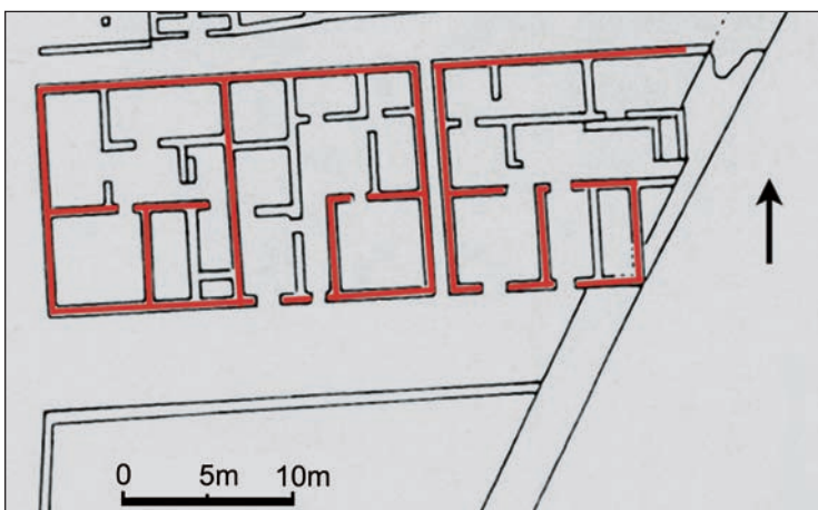
4. Ηράκλεια Μινώα, ανασκαμμένα σπίτια. Αν και το κάθε σπίτι έχει τη δική του διάταξη, οι παχύτεροι τοίχοι που φέρουν το μεγαλύτερο φορτίο (με κόκκινο χρώμα) βρίσκονται στην ίδια θέση σε κάθε σπίτι.
