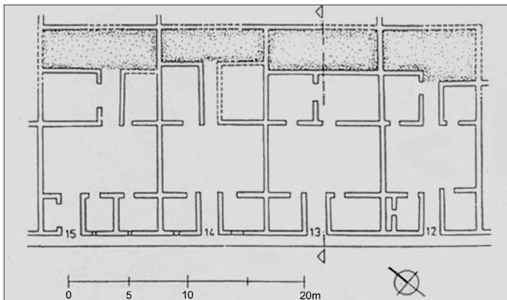
7. Πομπηία, αποκαταστημένες κατόψεις σπιτιών (Reg. I.11.12-15).
