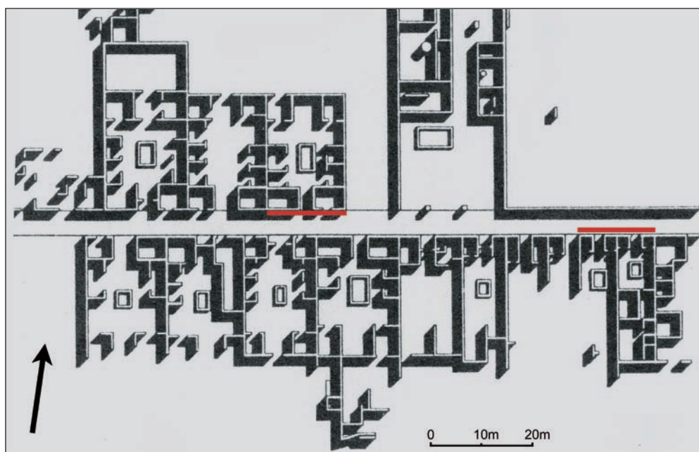
8. Φρεγγέλλες, αποκαταστημένη κάτοψη ενός ανασκαμμένου σπιτιού βορειανατολικά της Αγοράς.
