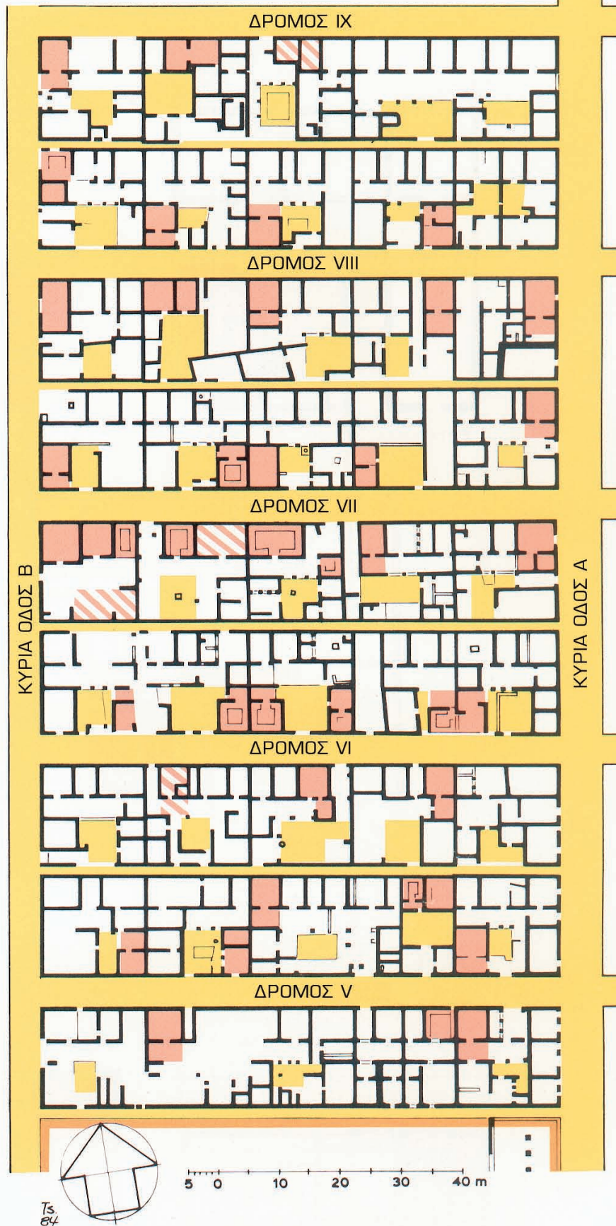
3. Όλυθος, σχεδιαστική αποτύπωση των ανασκαμμένων σπιτιών που παρουσιάζουν συνεχόμενους τοίχους στους άξονες από ανατολικά στα δυτικά.
